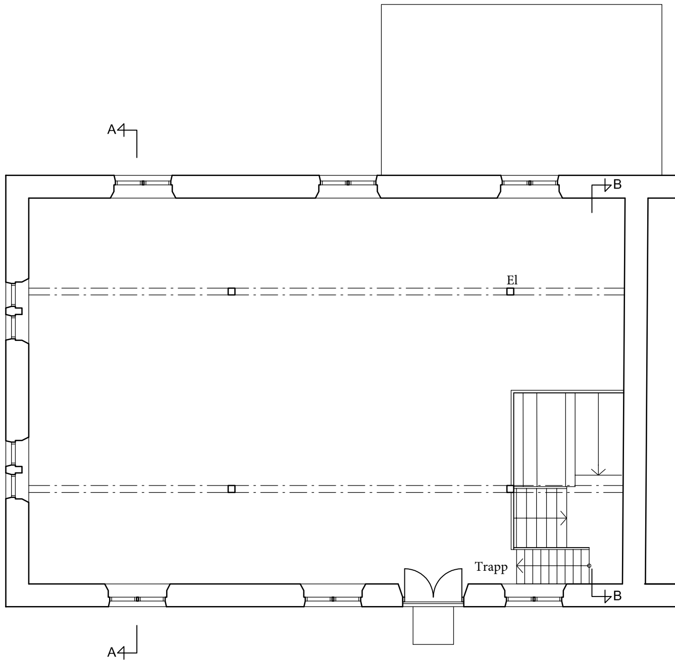
Plan ÖV, skala 1:100 (A4)
